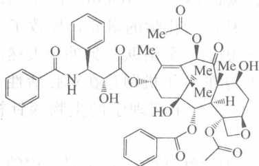
11 Paclitaxel (Taxol)
