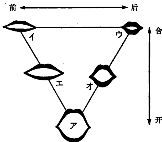
日语元音口形开合和发音示意图
