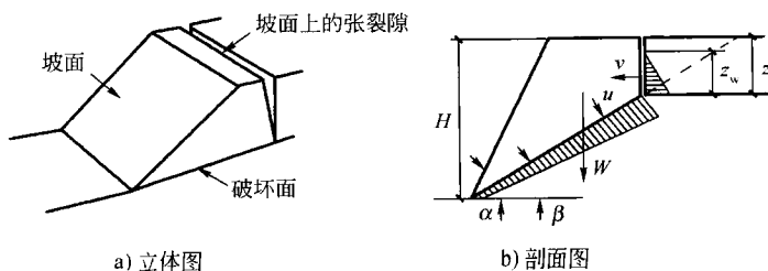
题 1-22 图 直线滑坡稳定系数计算
