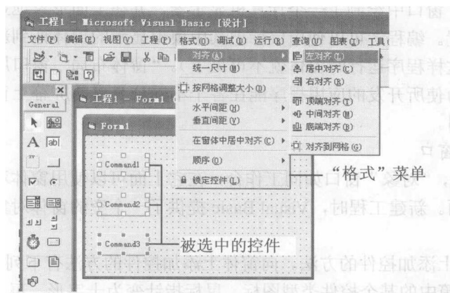
图 1-12 使用“格式”菜单对控件进行排布
