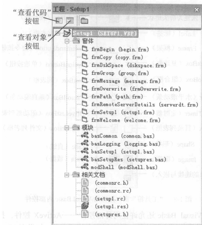
图 1-9 “工程”窗口
