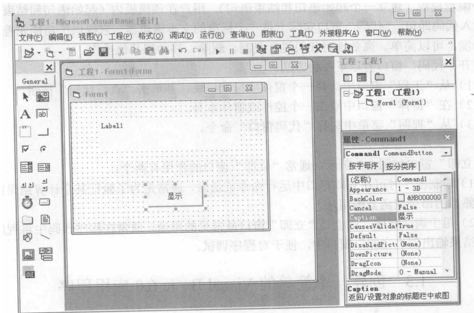
图 1-14 绘制好的控件及控件的属性列表
