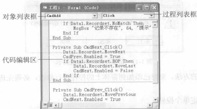
图 1-13 “代码”窗口
