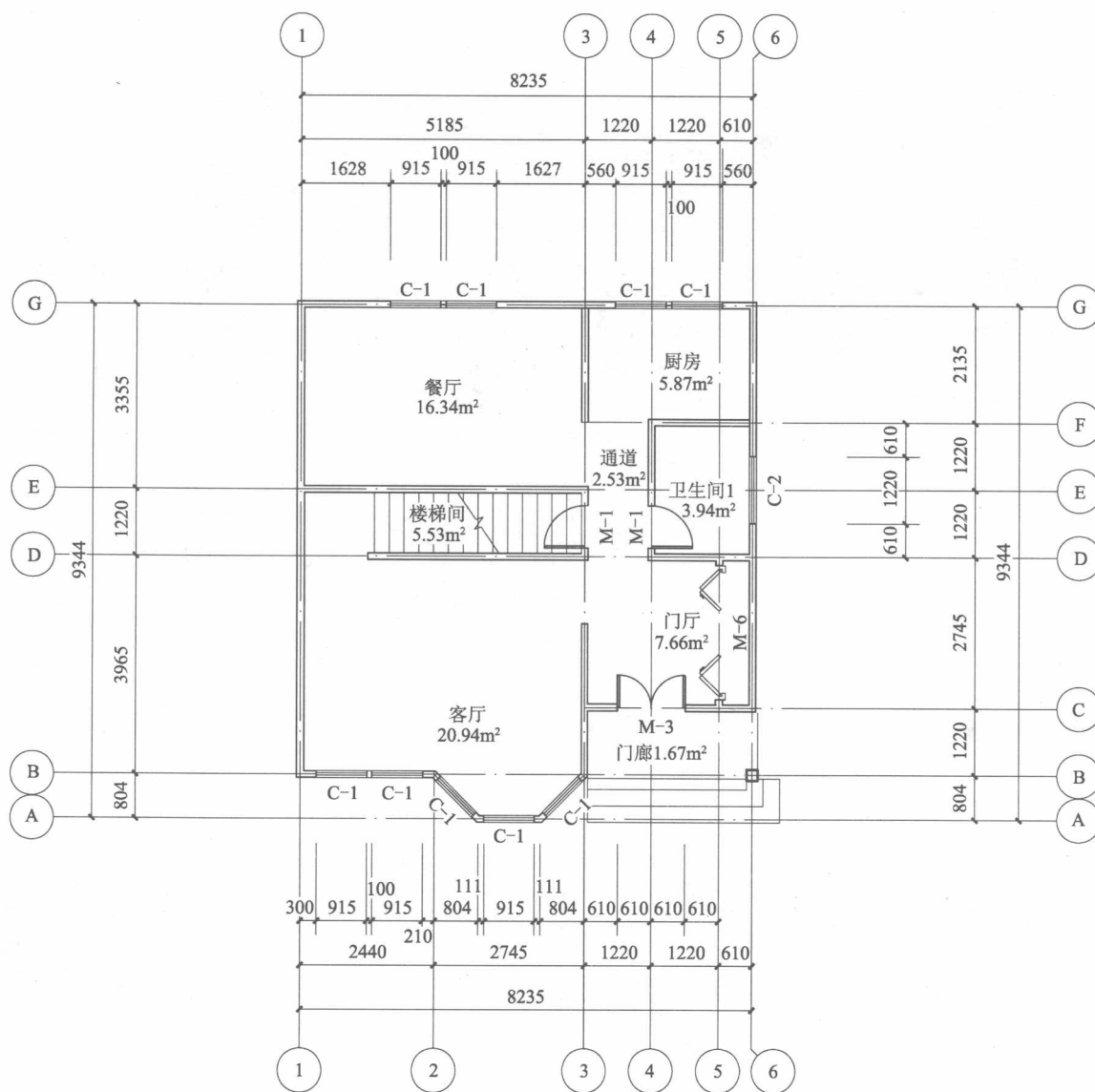
一层平面图
