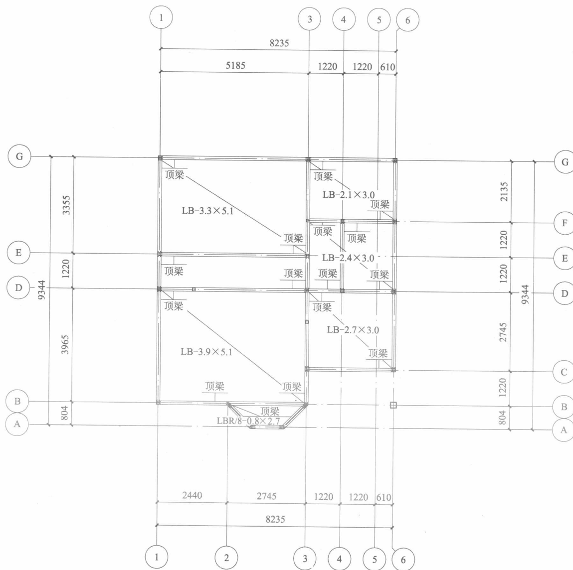
一层顶梁及楼板布置图
