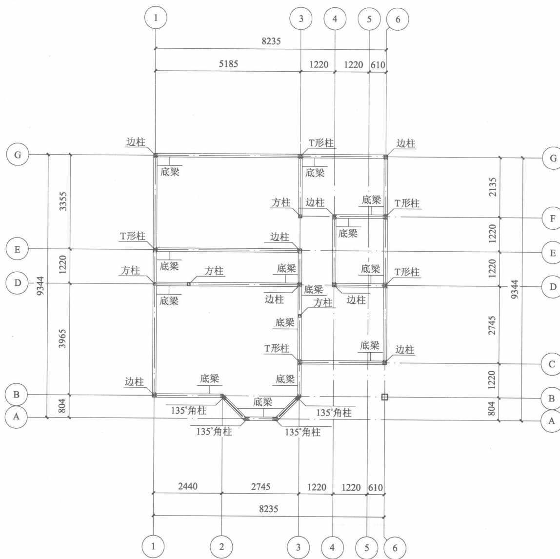
一层底梁及柱布置图
