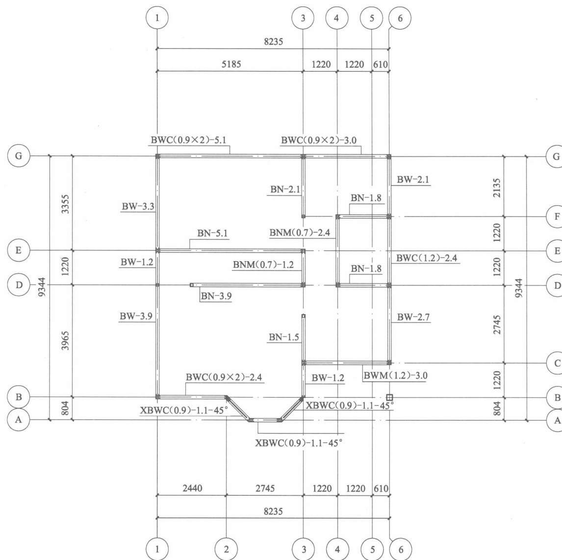
一层墙板布置图
