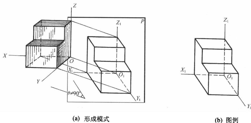
图1-10 斜轴测图
