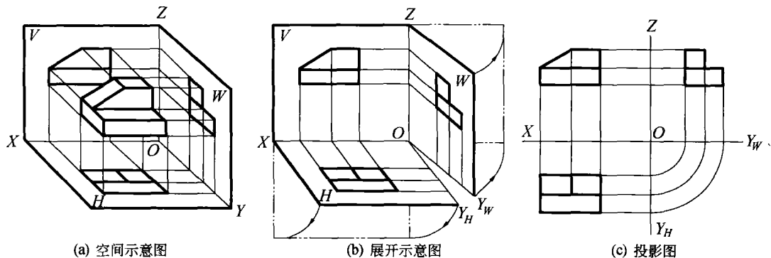
图1-8 立体的三面投影
