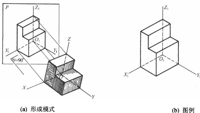
图1-9 正轴测图
