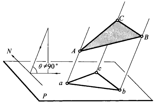
(b) 斜投影法
