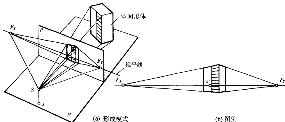
图 1-11 透视图
