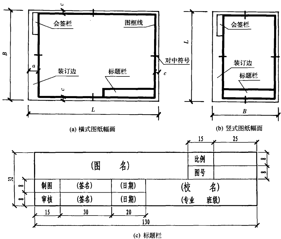
图 2-1 图纸幅面、格式及标题栏
