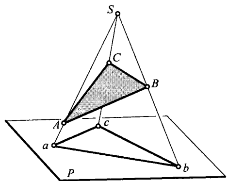
图 1-2 中心投影法
