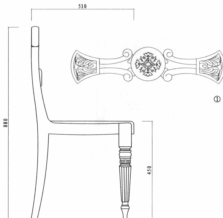
左视图 left view
