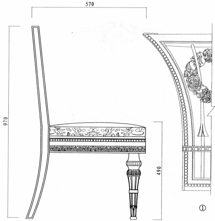
左视图 left view
