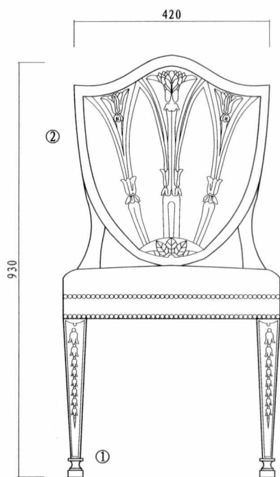
主视图 front view
