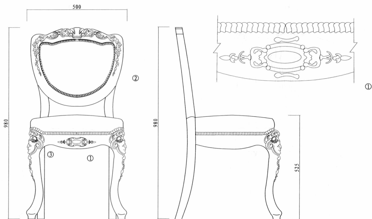
主视图 front view
