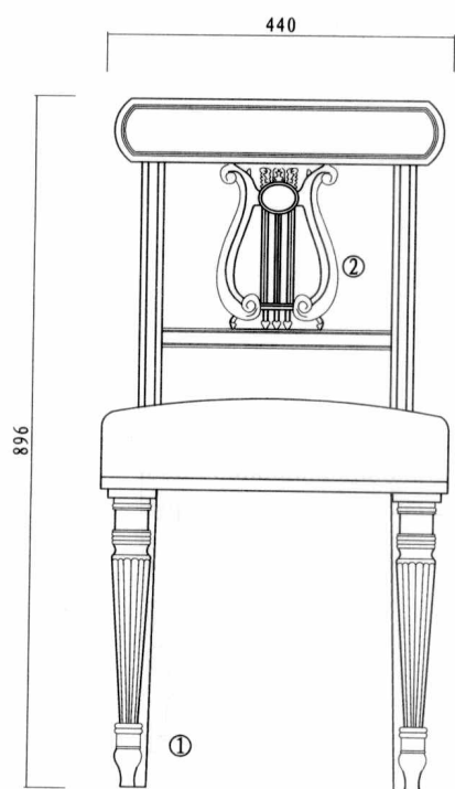
主视图 front view
