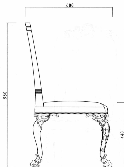
左视图 left view
