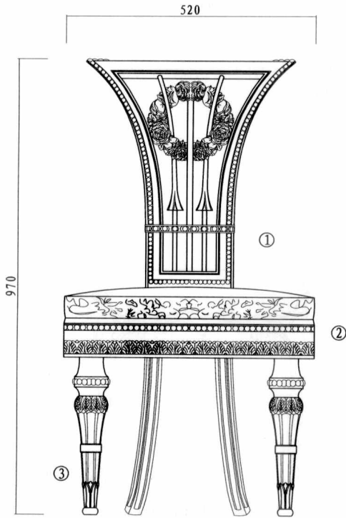
主视图 front view
