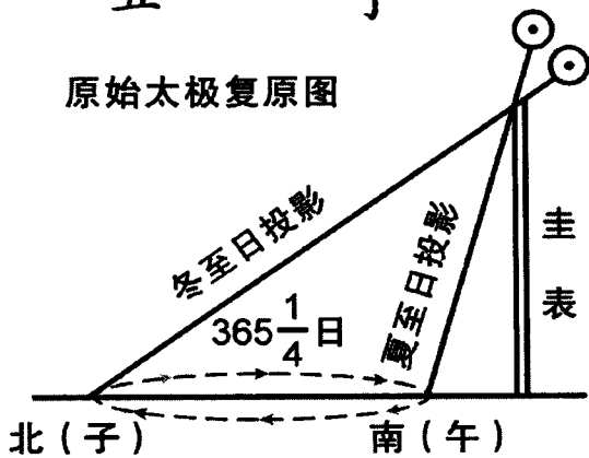
伏羲测量四季变化与二十四节气变化图
