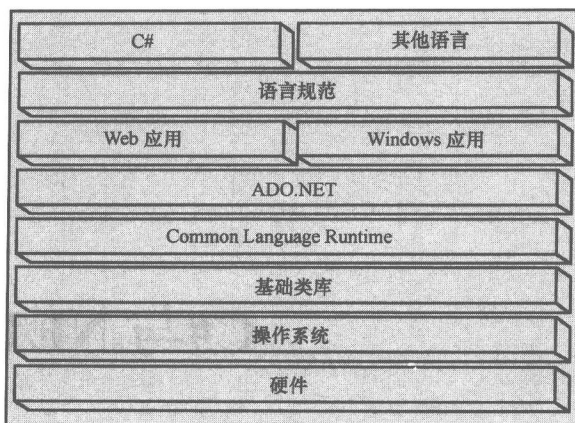
图 1-1 .NET 框架基本结构
