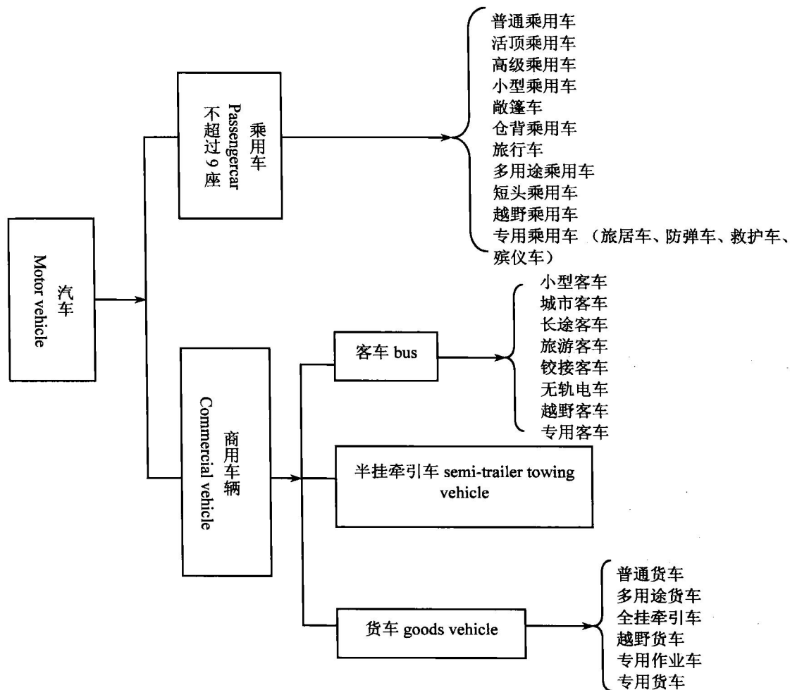
图 1-1 汽车的分类 (根据 GB/T3730.1—2001 整理)
