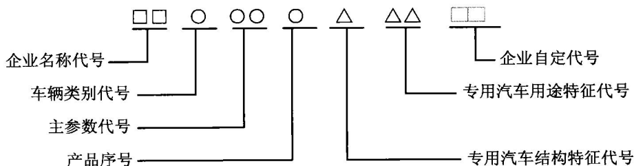
图 1-3 专用汽车型号组成示意图
