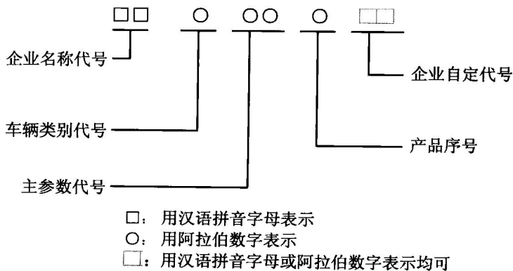
图 1-2 汽车型号组成示意图
