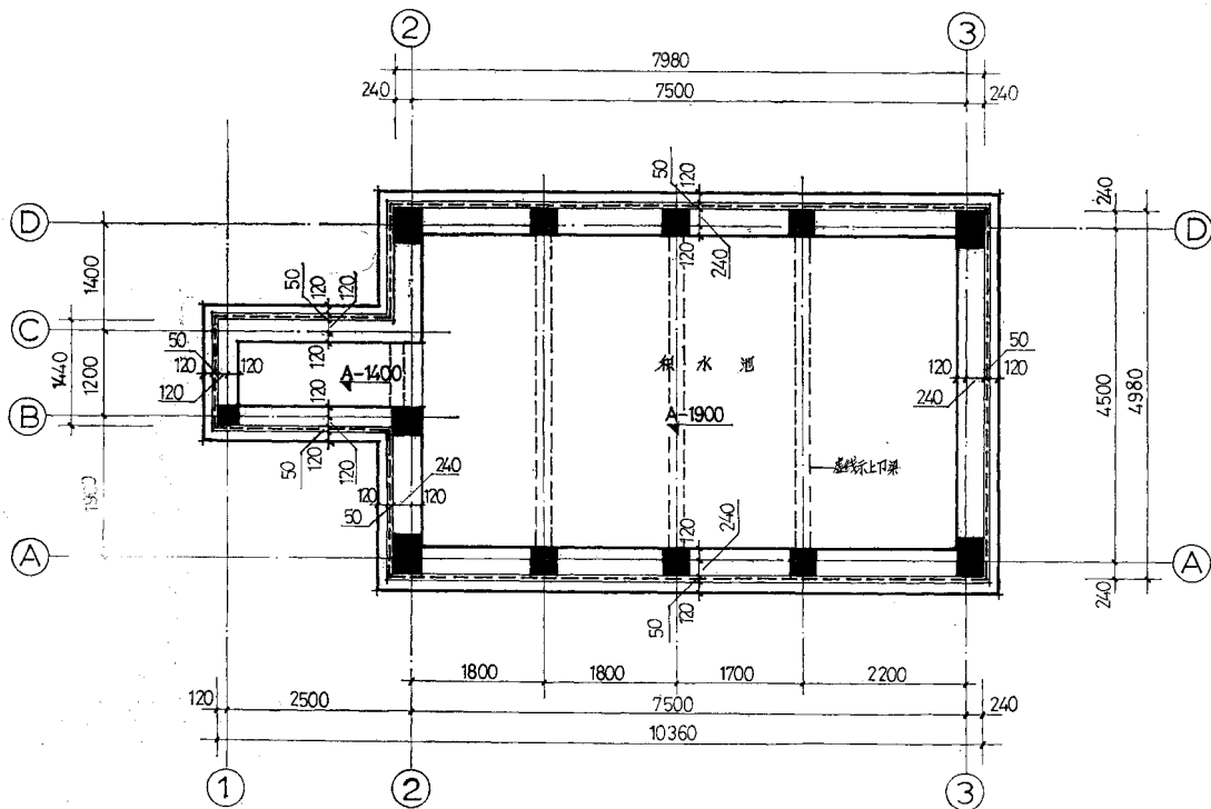
积水池平面 1:50
