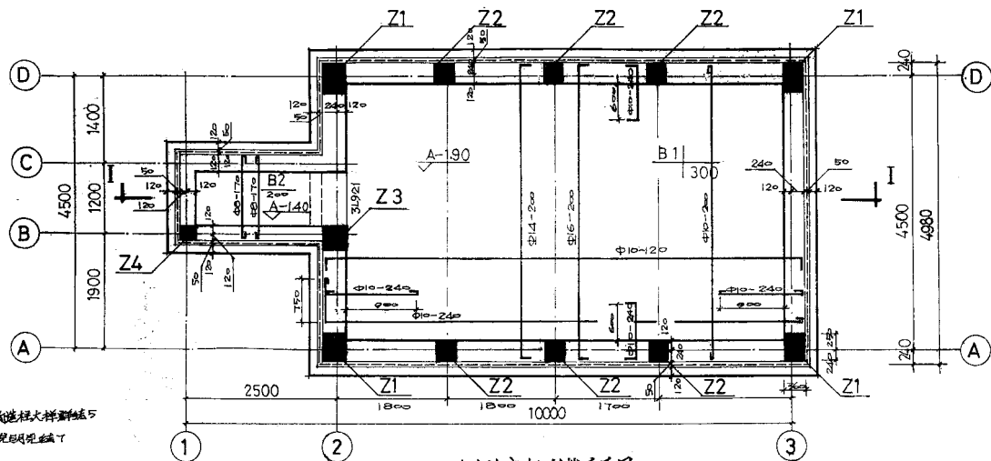
积水池底板配筋平面图 1:50
