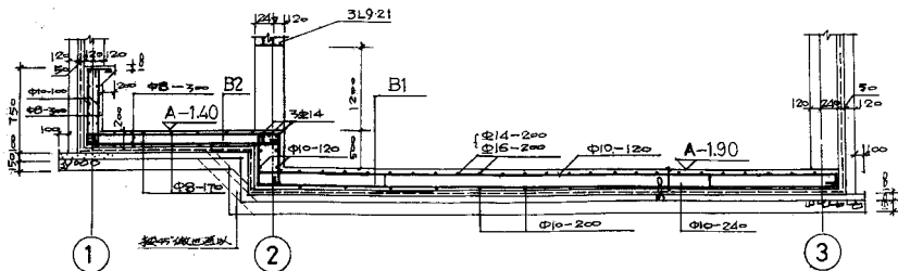
积水池底板配筋剖面图 1:50 (I-I)
