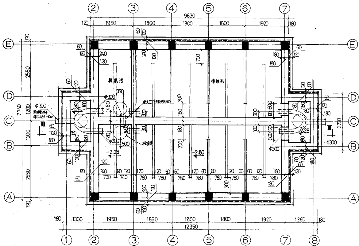
投氯、接触池平面 1:50
