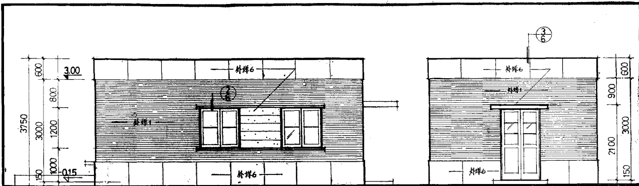
侧立面 1:50
