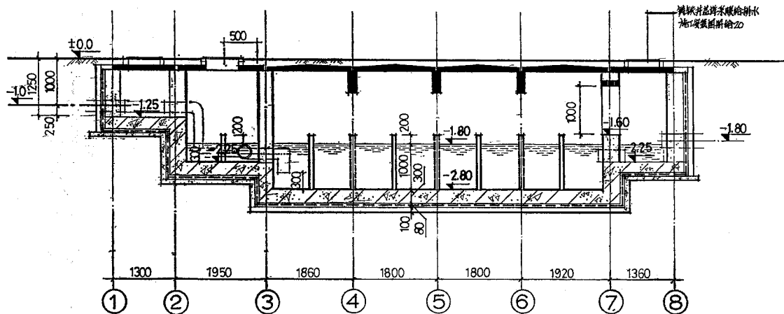
II—II 剖面 1:50
