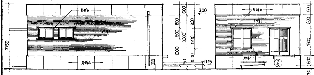
侧立面 1:50
