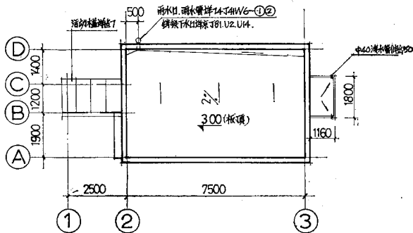
屋顶平面 1:100
