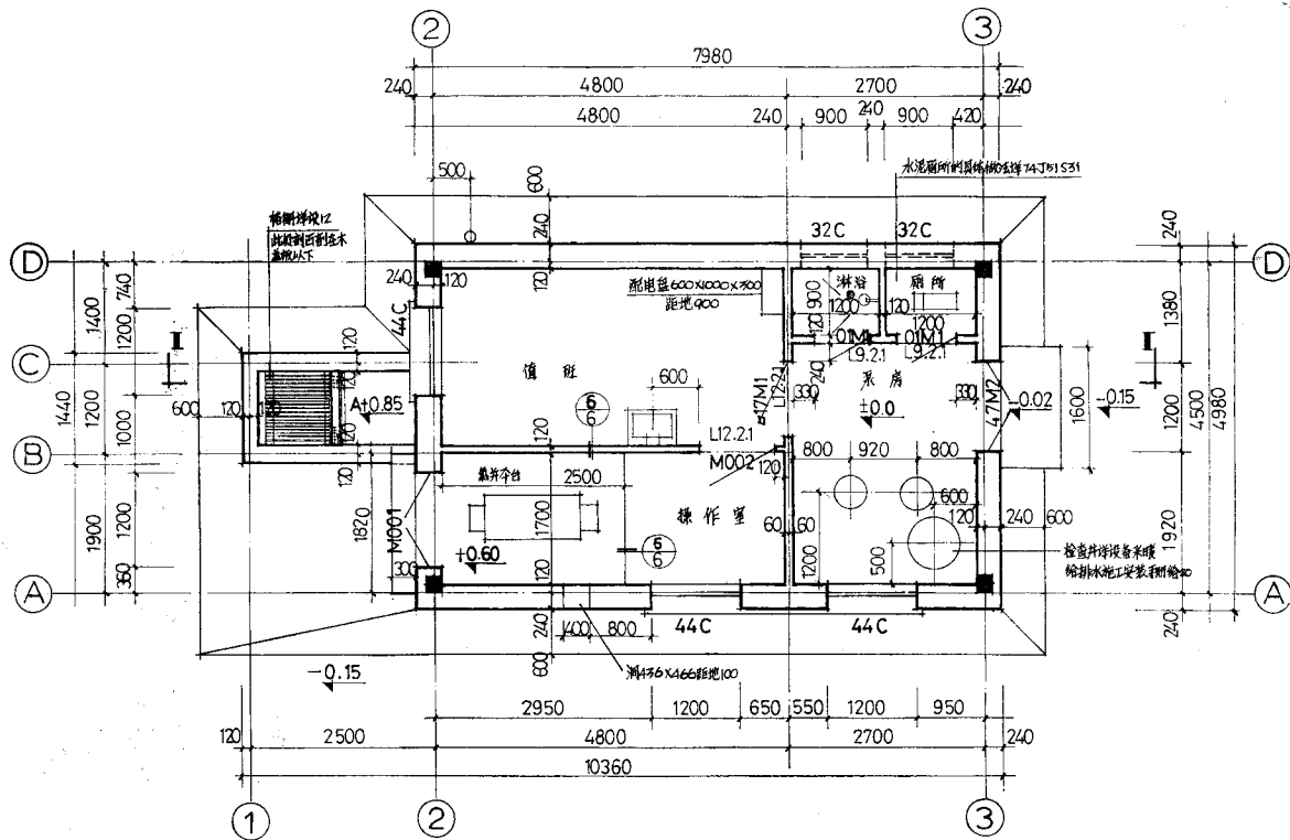
泵房操作室平面 1:50
