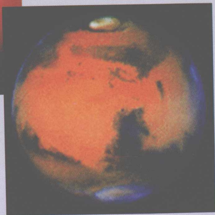
火星
