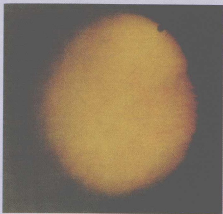
金星凌日
