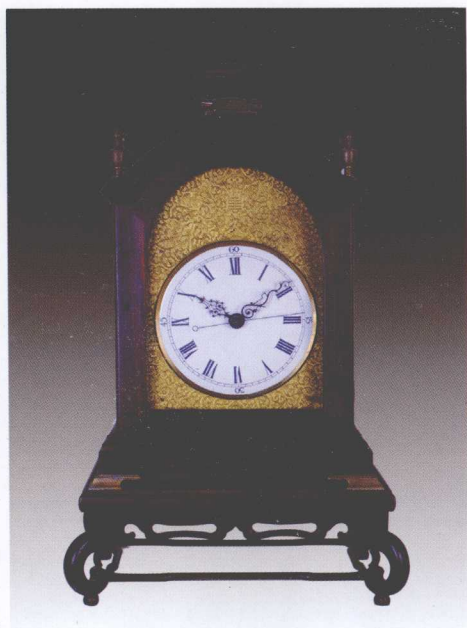
中国产2号广式钟 19世纪晚期。高540毫米，宽315毫米，厚210毫米。白搪瓷表盘，黑罗马数字，烤蓝花时刻针，细长秒针。铜鎏金五福捧寿面板，优质老红木外壳。机器为单铃，打点不报刻。
