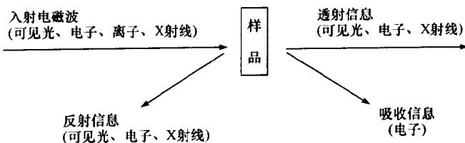
图 1.3 样品特征物理信息示意图
