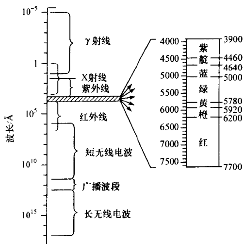
图 2.1 电磁波谱
