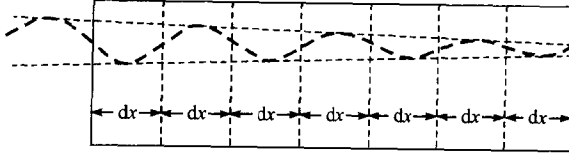
图 2.4 晶体对光的吸收
