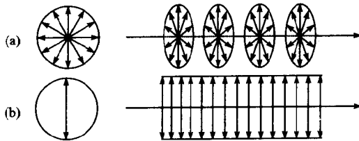
图 2.2 自然光和偏振光振动示意图 (a) 自然光;(b) 偏振光
