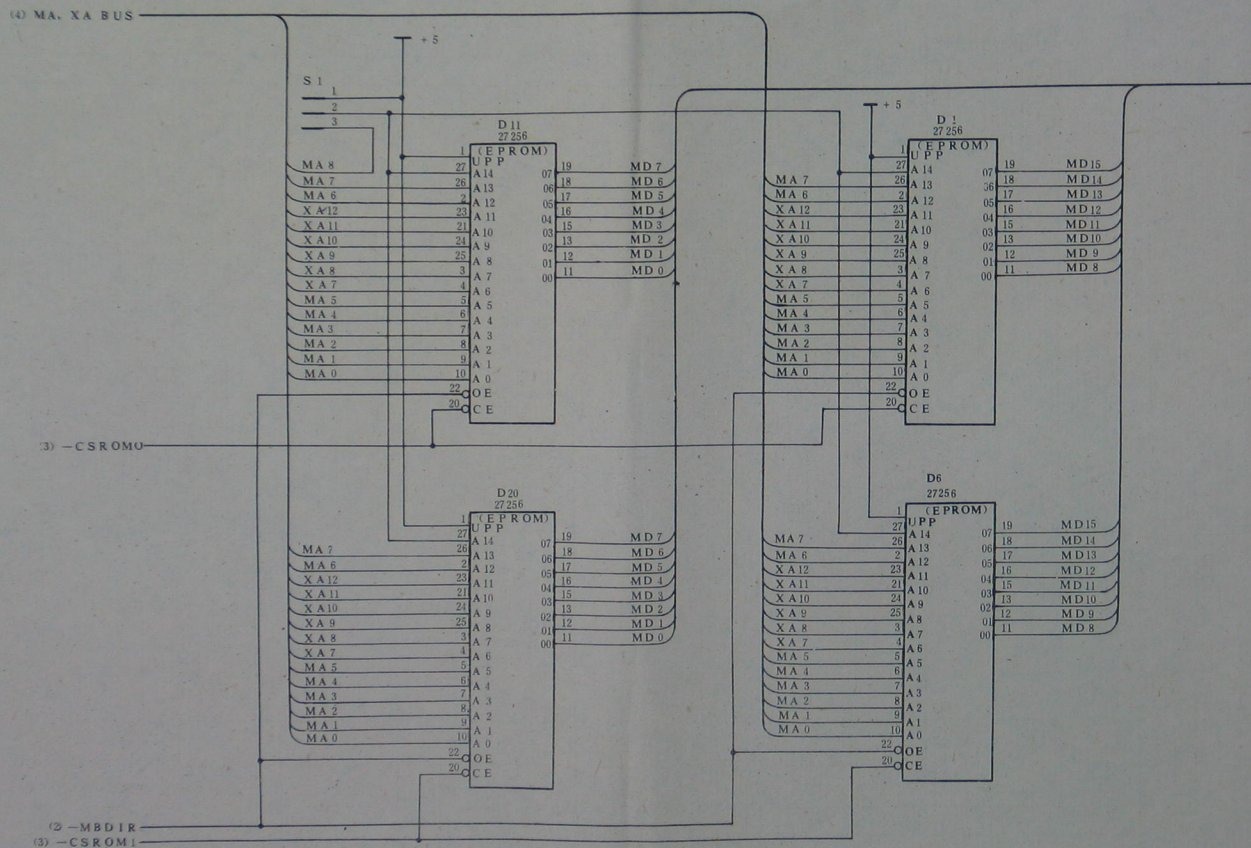
系统板逻辑电路(2)
