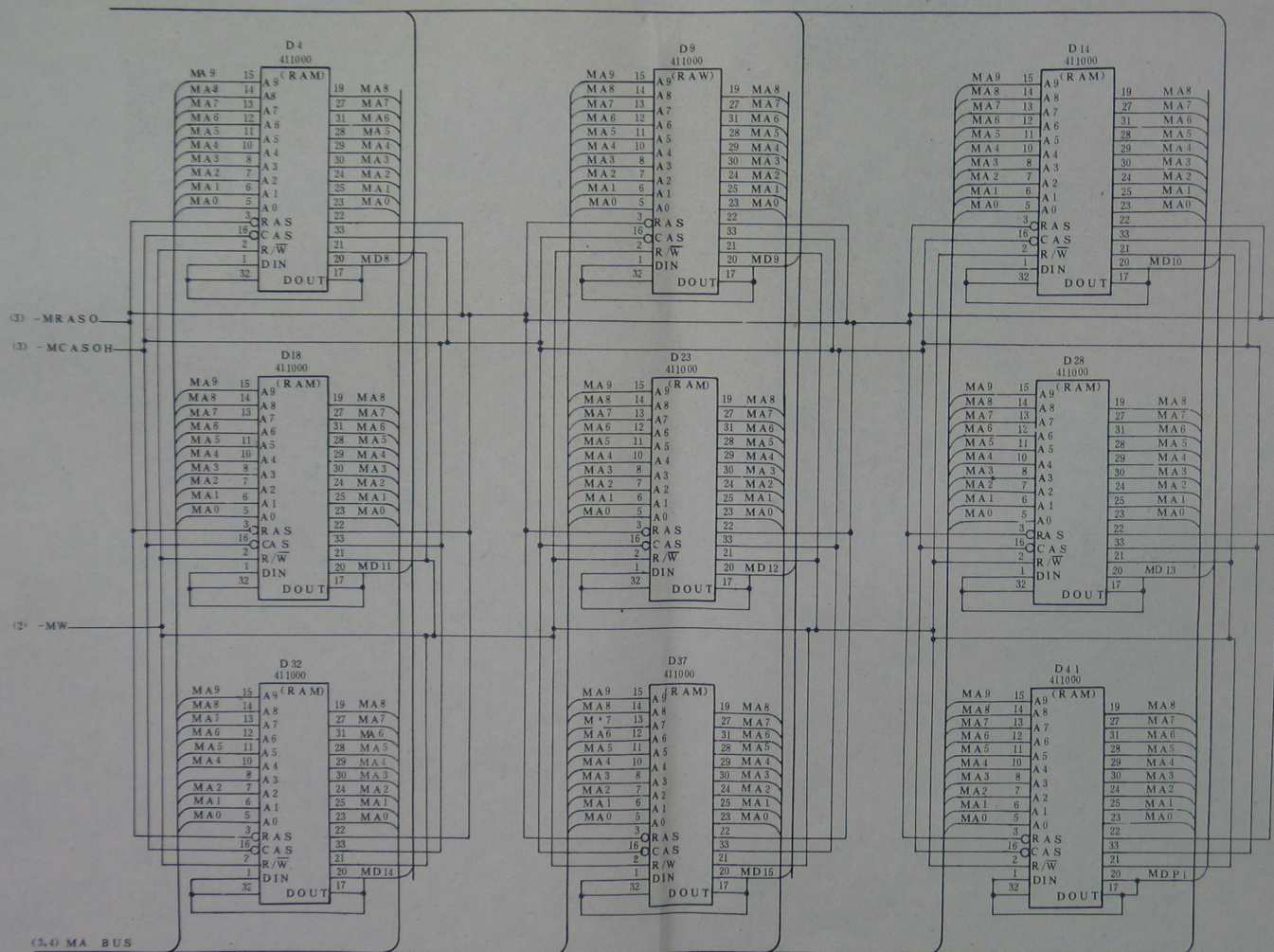
系统板逻辑电路 (9)
