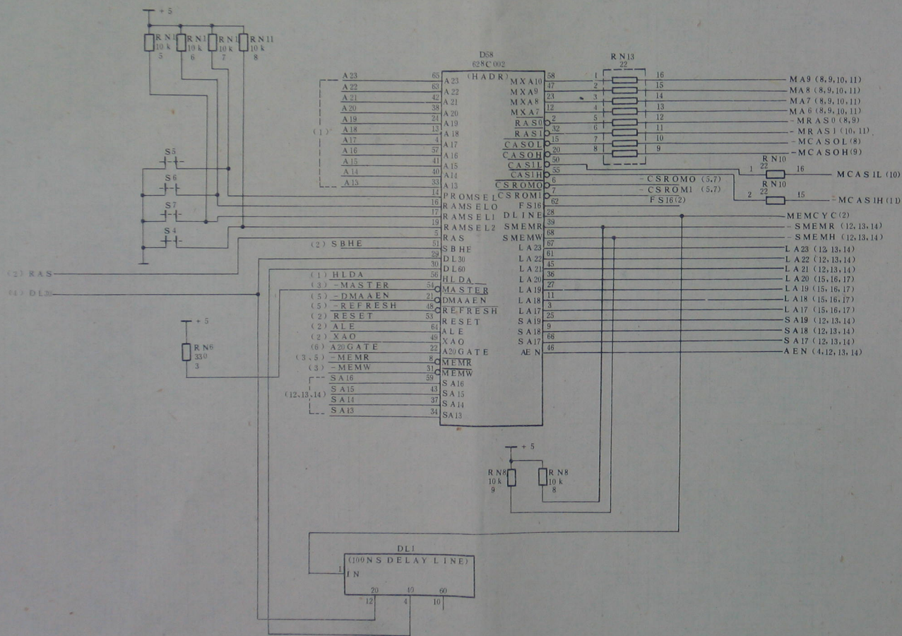
系统板逻辑电路 (4)
