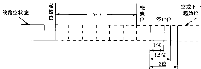
图 1-9 异步传输
