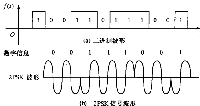
图 1-3 数字信号波形
