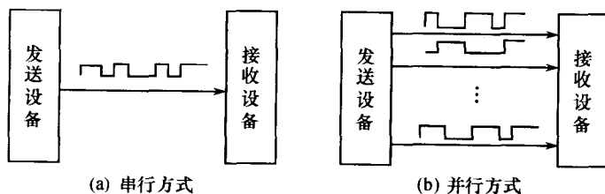
图 1-8 串行和并行传输方式
