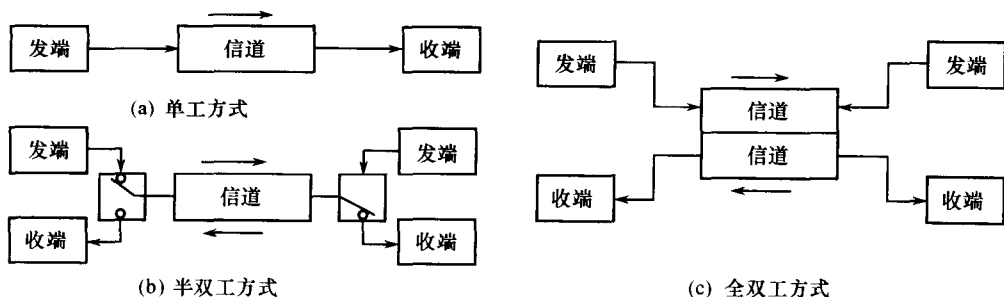
图 1-7 通信方式示意图
