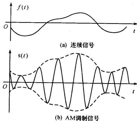
图 1-2 模拟信号波形
