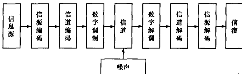
图 1-5 数字通信系统模型
