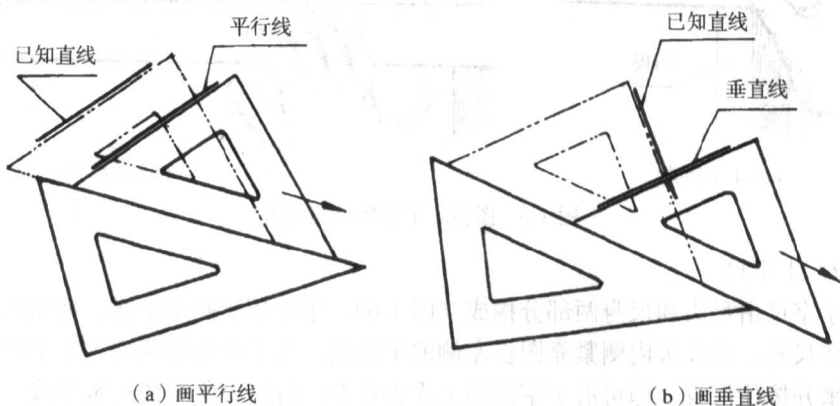
图 1-8 将两块三角板配合使用
