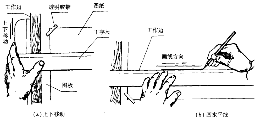
图 1-6 图板、丁字尺及其使用
