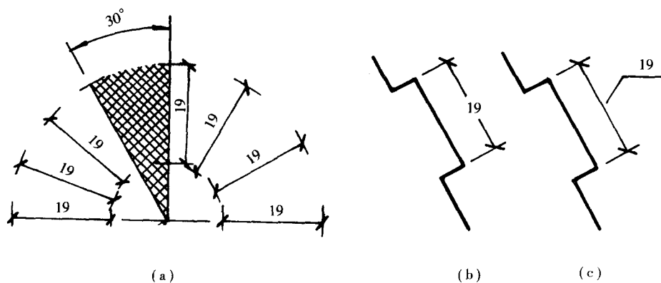
图 1-4 线性尺寸数字的注写方向
