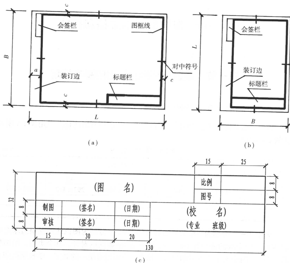
图 1-1 图纸幅面、格式及标题栏
