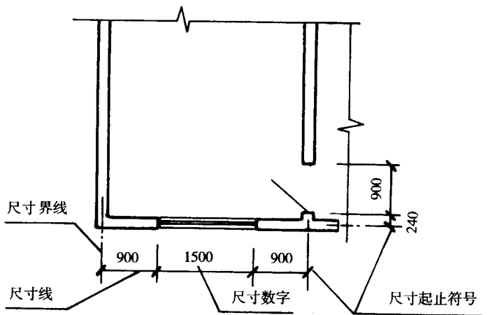
图 1-3 尺寸标注的基本形式和组成
