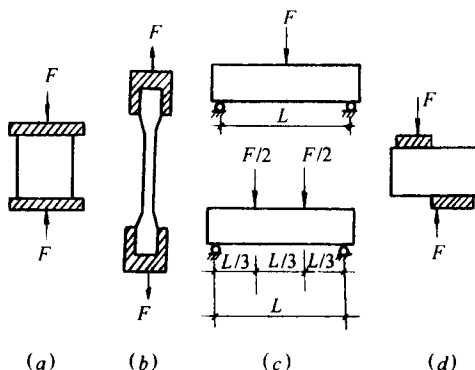
图 20-2 材料受力示意图
