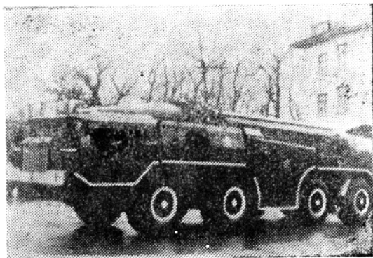
苏飞毛腿B导弹。射程可达300公里,发射全重6300公斤,可装炸药900余公斤或核弹头。
