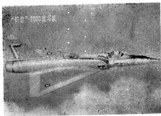
法“幻影”—2000战斗机。装有2门30毫米机炮可挂4枚导弹。作战半径650公里。
