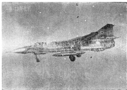
苏米格—23歼击机。装有1门23毫米双管机炮，可挂4枚空对空导弹或炸弹、火箭，作战半径1160公里。
