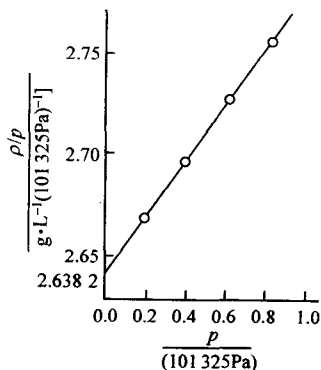
图 1-2 0^\circ\text{C} 时三甲胺的 \frac{\rho}{p} - p 图
