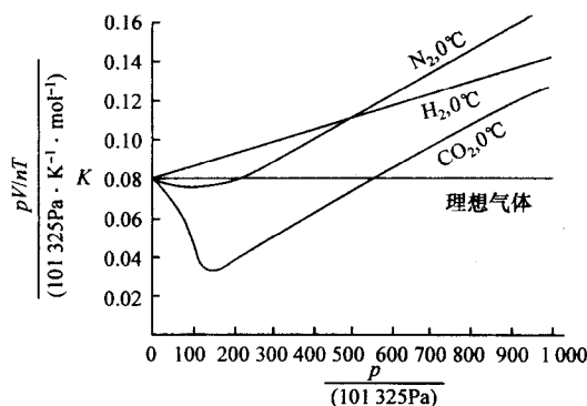
图 1-1 外推法求 R 值
