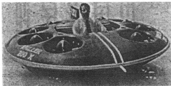
天才莫勒对 M200X 进行试验
