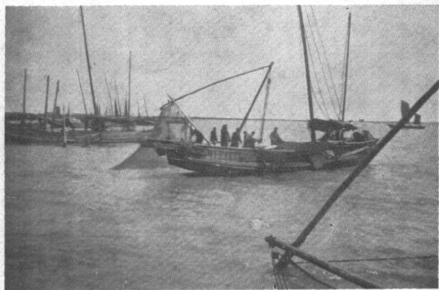
吳淞口銀魚挑網漁船放網情形
