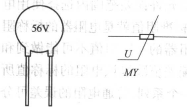
图 2-5 压敏电阻的外形及符号
