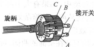
大电位器
