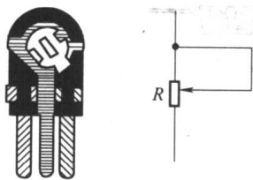
图 2-3 半可变电阻的外形及符号
