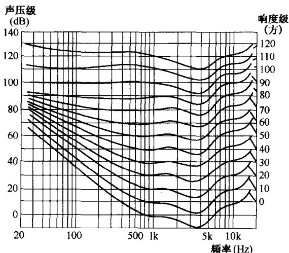
图 1-5 人耳的等响度曲线
