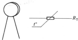
图 2-4 热敏电阻的外形及符号
