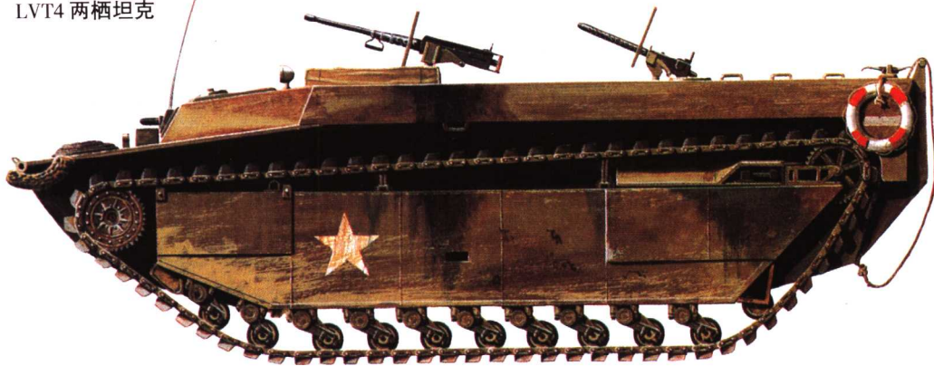
LVT4 两栖坦克
