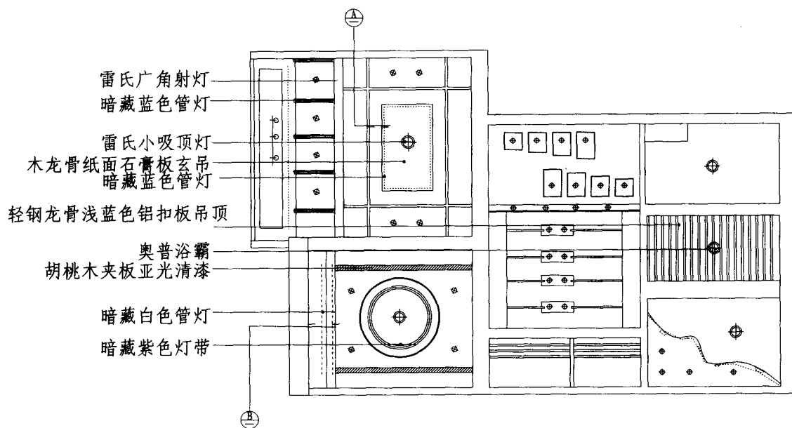
平面图
