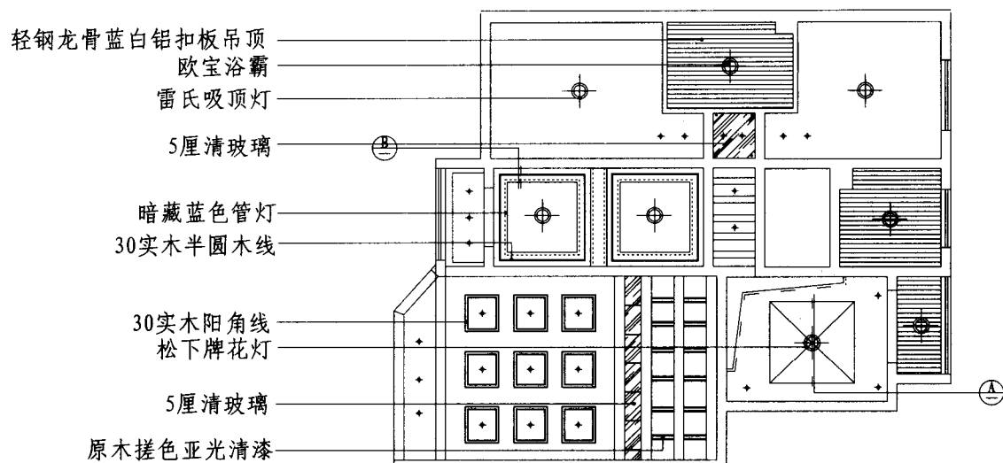
平面图
