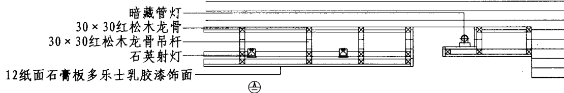
节点图
