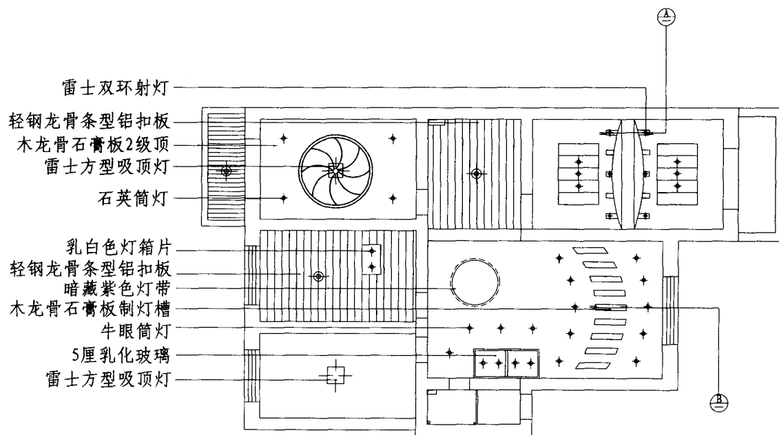
平面图
