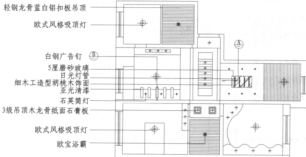
平面图
