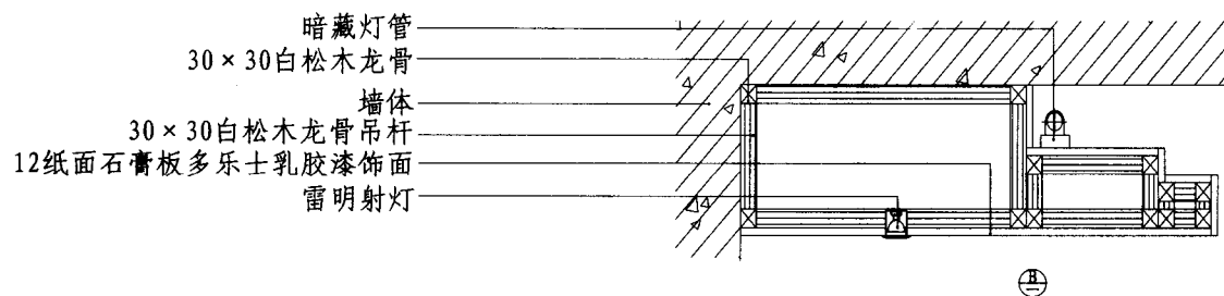
平面图
