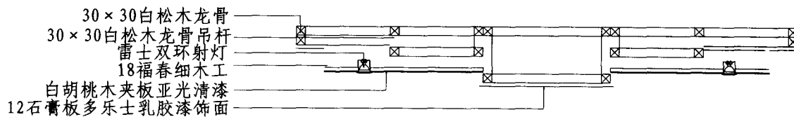
节点图
