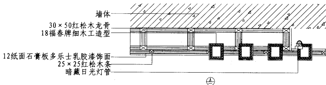
平面图
