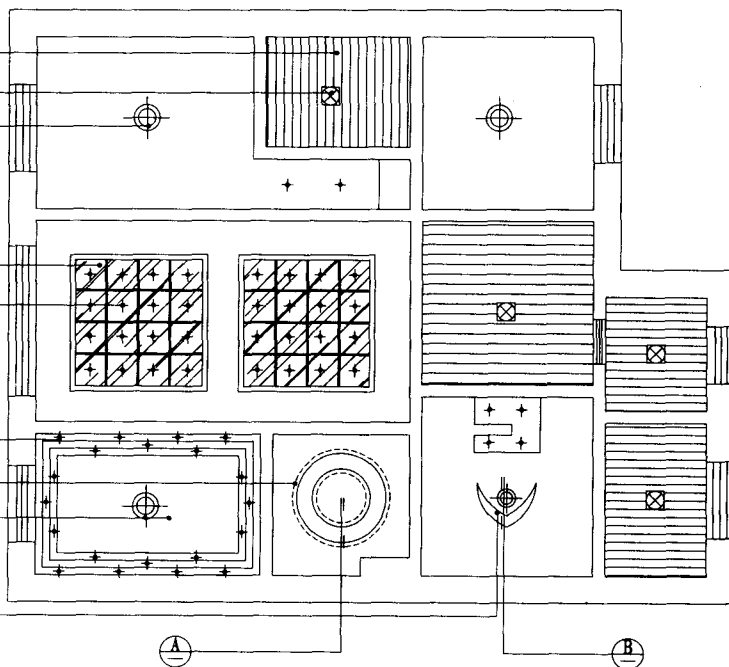
平面图
