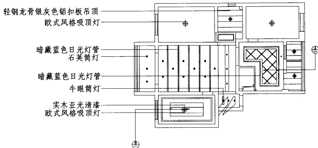
平面图
