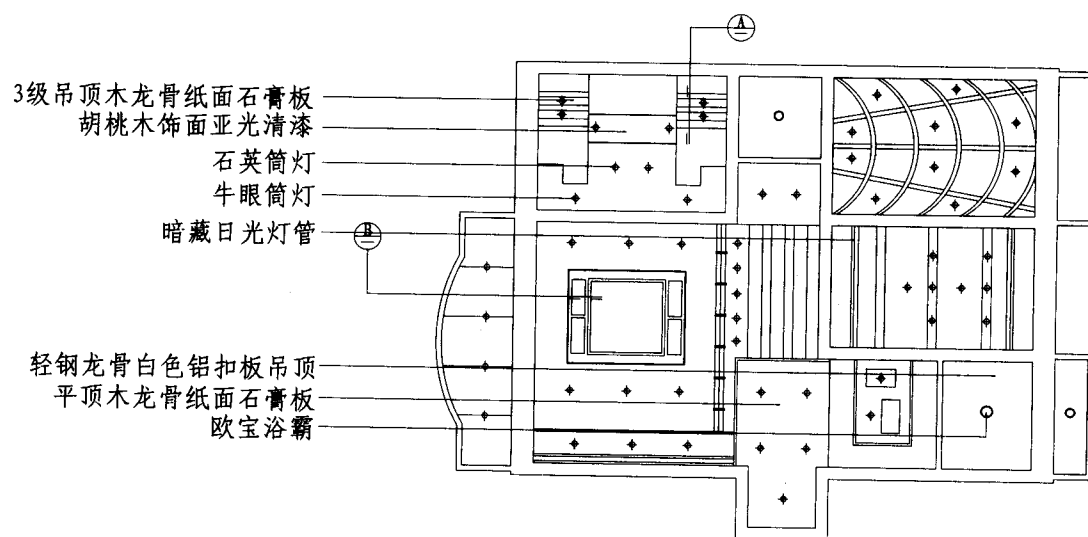
平面图
