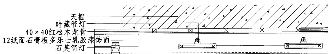
平面图
