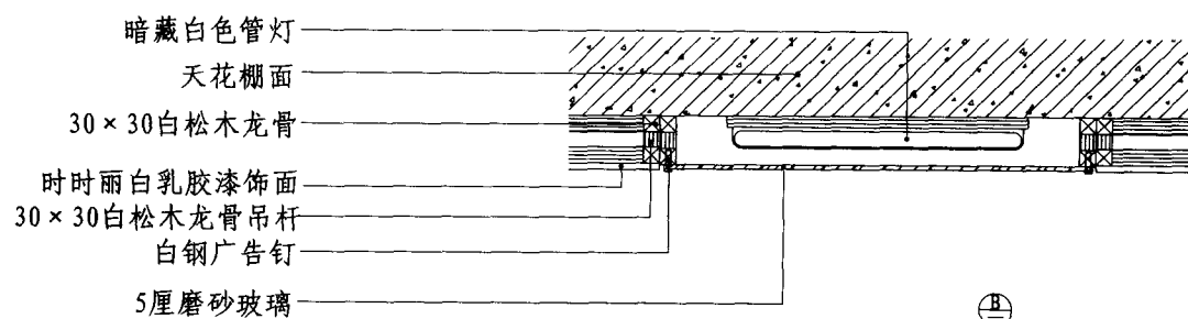
节点图
