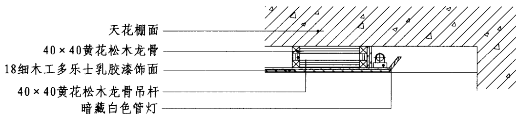
节点图
