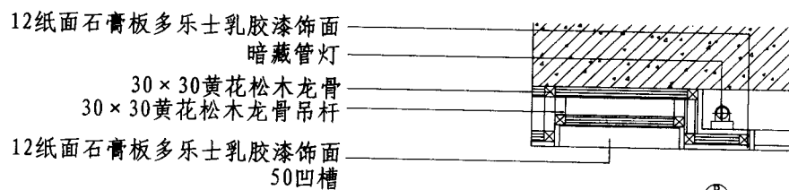
节点图
