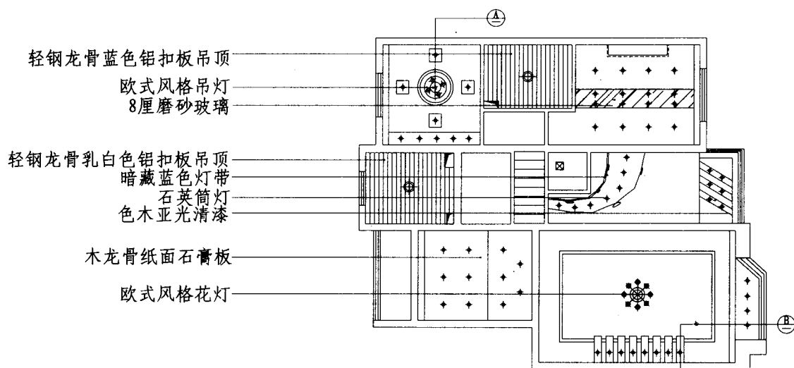
平面图
