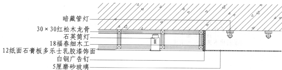
节点图
