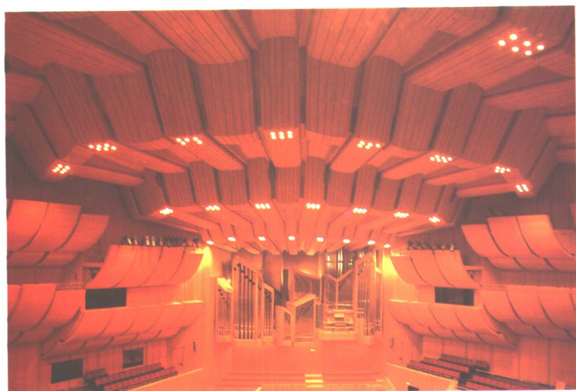
图 2-117 德国慕尼黑音乐厅的声学处理
