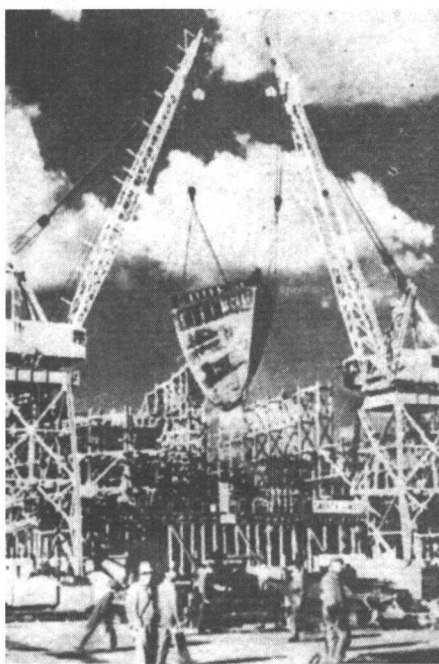
▲加州威尔明顿 (Wilmington) 造船厂的生产现场。这是运送放假船员的船(Liberty)舷的顶端部分的制作材料被高高吊起来的情景。大规模建造这样的船只船体都是焊接起来的,而不是铆在一起的,因此可以节省大量时间、人力和负重。所有在美国建造的英国船只都将采取焊接的方法。
