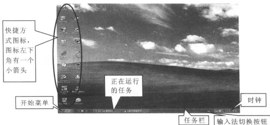
图 1-1 Windows 2000 的桌面
