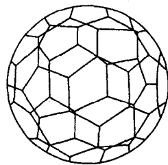
图 1-4 富勒烯
