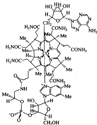
图 1-2 维生素 B 12
