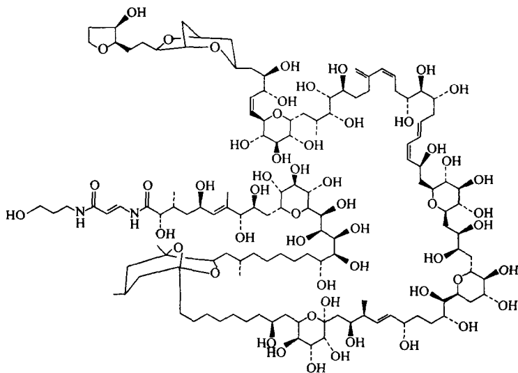
图 1-3 海葵毒素
