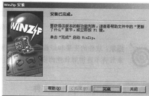
图 1.8 安装完成
