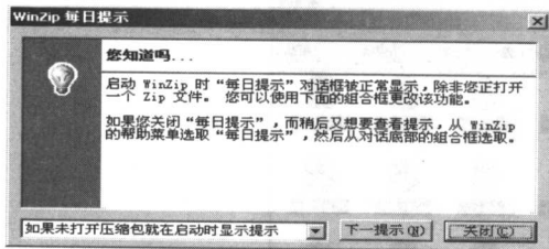
图 1.9 每日提示
