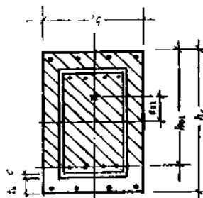
图 3.3.3 插入式柱连接处截面有效高度
