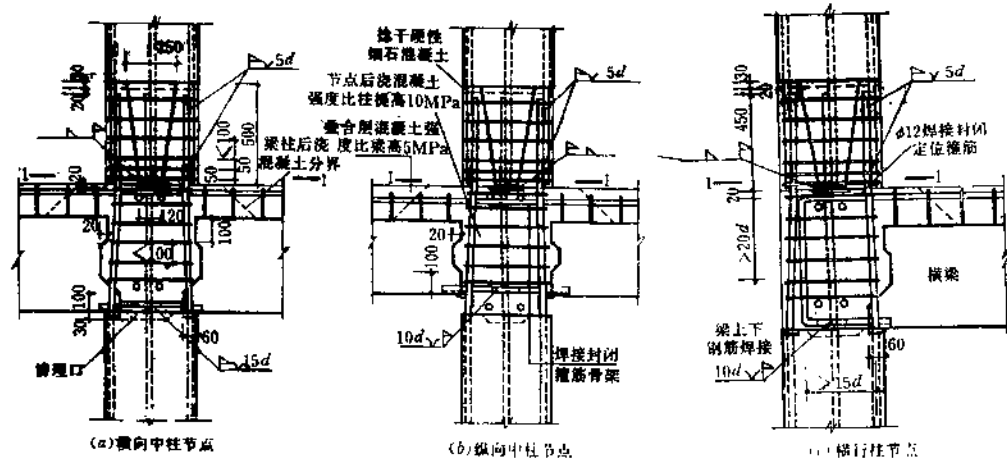
图 4.4.1-1 整浇式节点 (A型构造)
