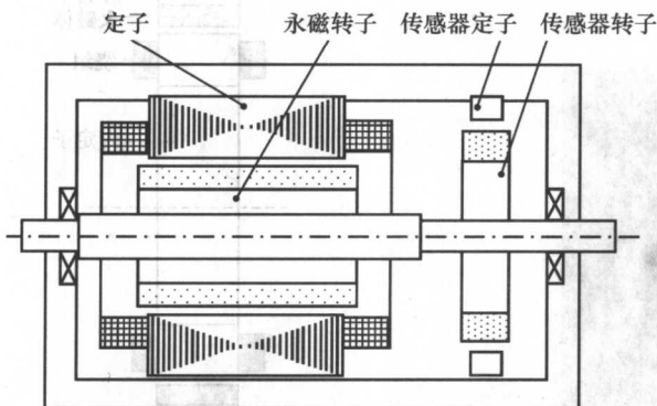
(a) 结构示意图
