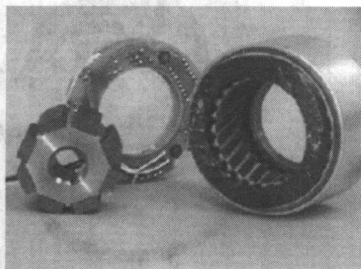
(b) 定转子实际结构
