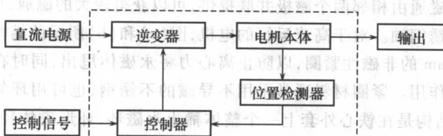
图 1-1 无刷直流电动机系统的组成
