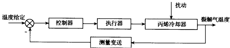
图 1.4 丙烯冷却器温度控制系统方框图
