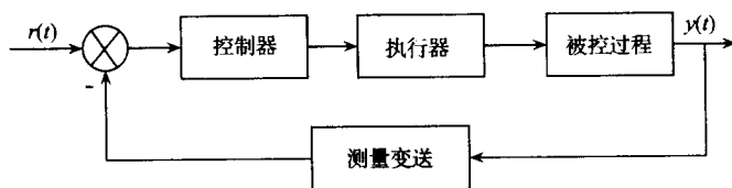
图 0.1 过程控制系统的一般结构
