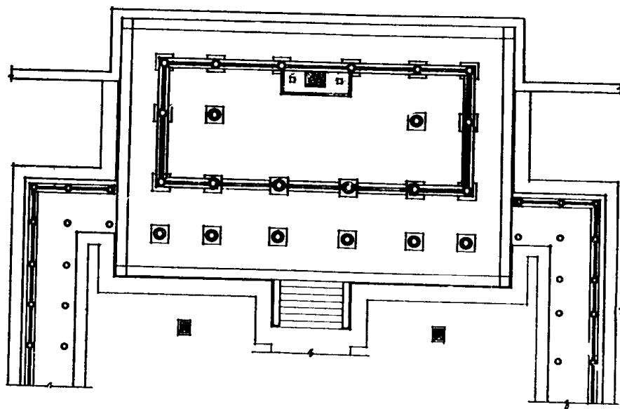
揚州·鑑真大和尚紀念堂平面圖 1 0.5 0 1 2 3 4 5m
