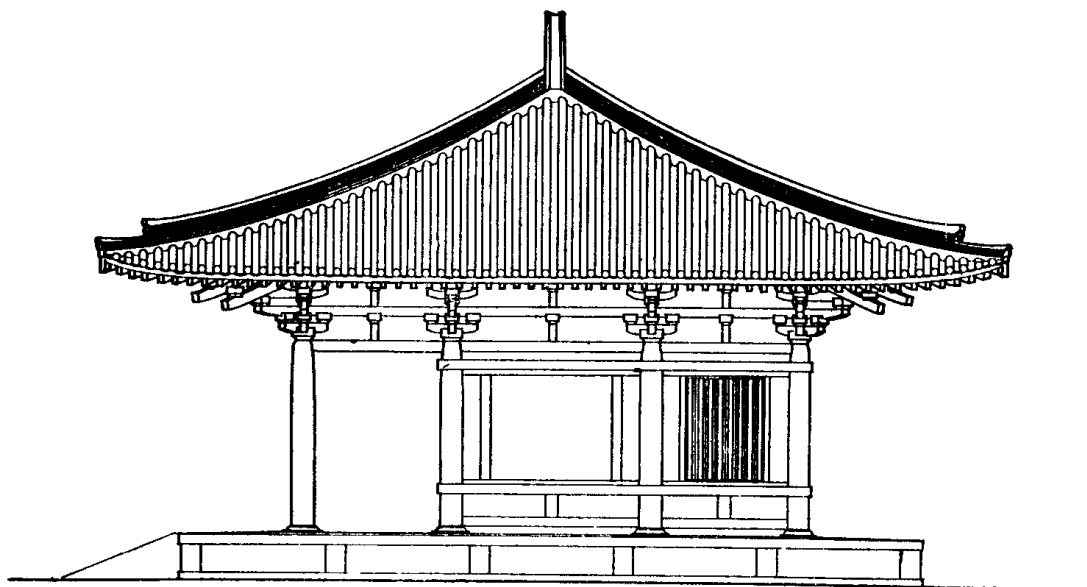
揚州 鑑真大和尚紀念堂側面圖 1 0.5 0 1 2m 图版六
