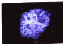
不灭的原子
