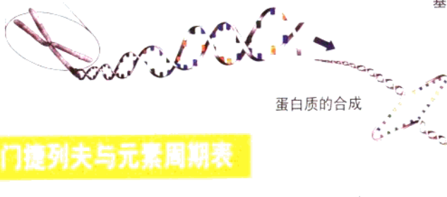
人的染色体
