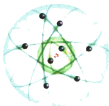
质子和中子
