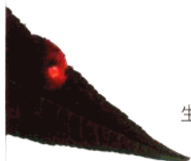
巴基球形的碳
