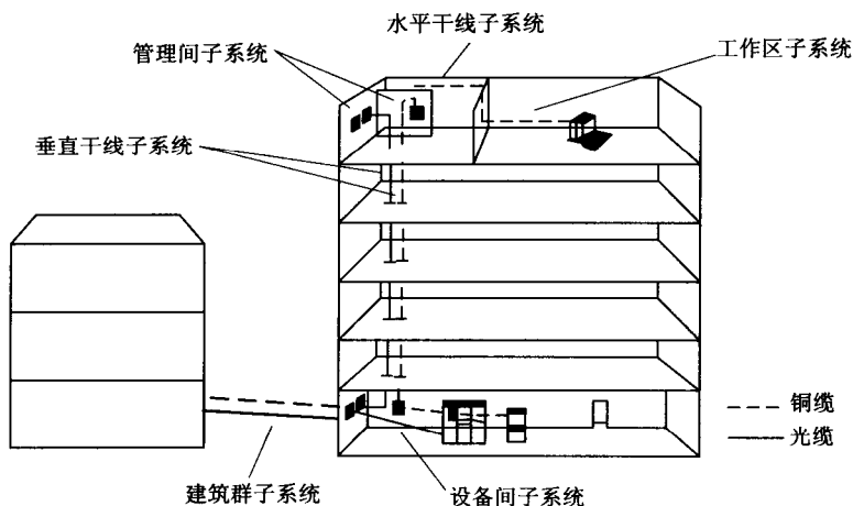
图 1.1 综合布线系统结构
