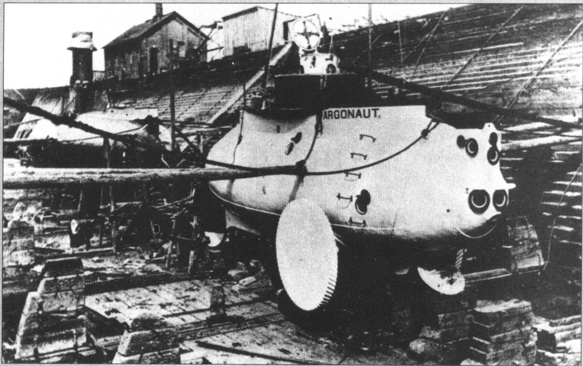
1897年，“阿尔戈英雄”号的建造工作在巴尔的摩基本完成。莱克将他变卖自己股份所得的2500美金用于这艘潜艇的建造。
