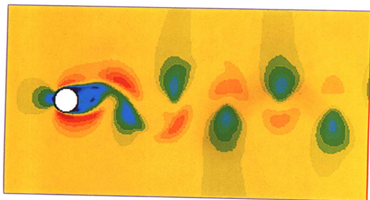
图6 卡曼涡街数值模拟照片
