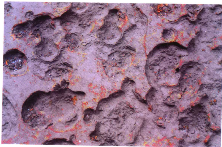
图5 换热器壳体表面 腐蚀失效照片
