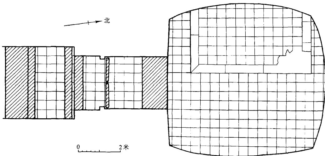
图 3 墓葬甬道、墓室平面图
