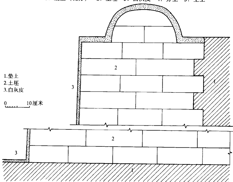
图7 墓道壁剖面示意图
