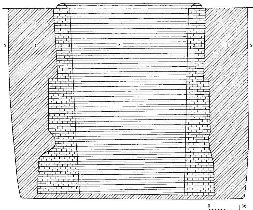
图6 墓道横剖面图
