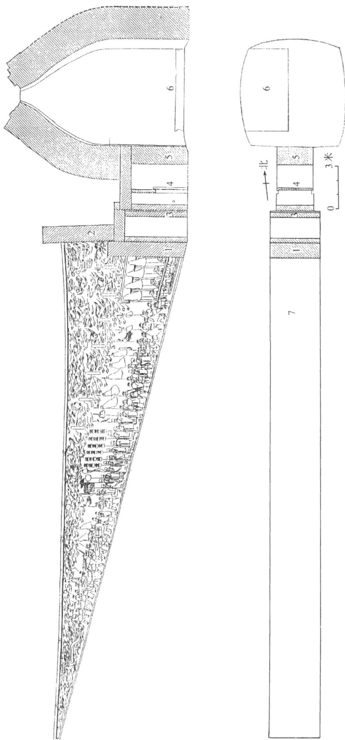
图 4A 墓葬平、剖面示意图 1. 南封墙 2. 门墙 3. 中封墙 4. 石门 5. 北封墙 6. 棺床 7. 墓道
