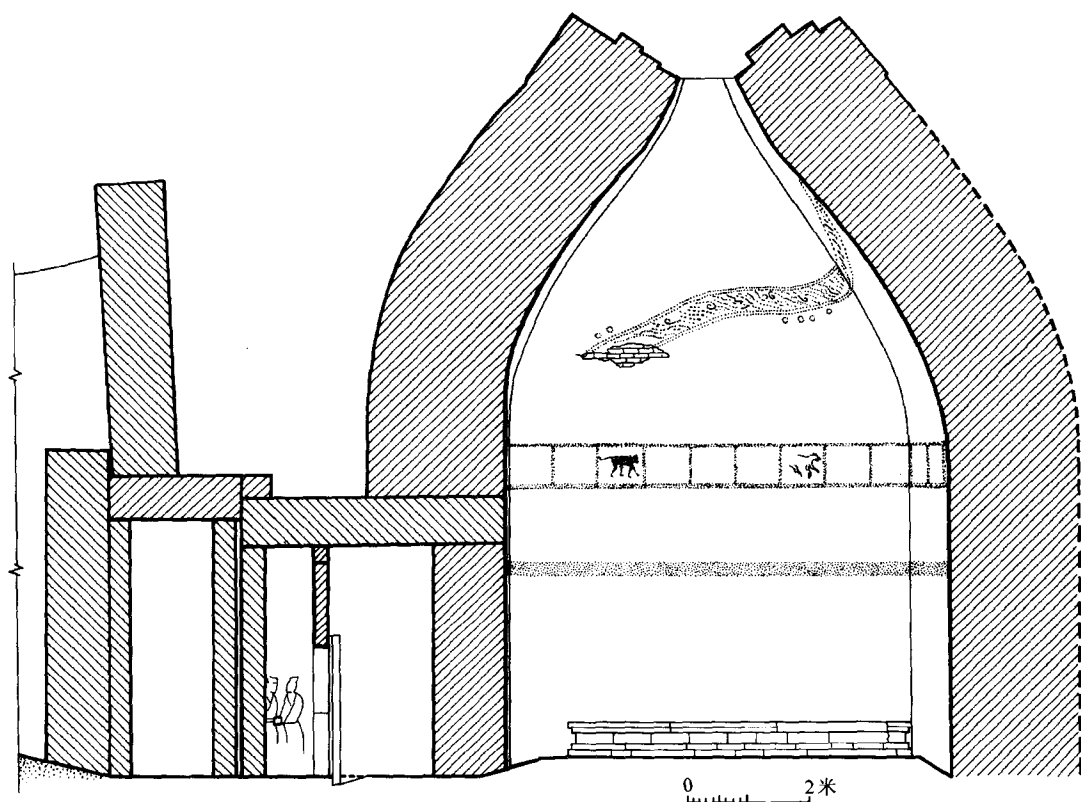
图 4B 墓室、甬道剖视图
