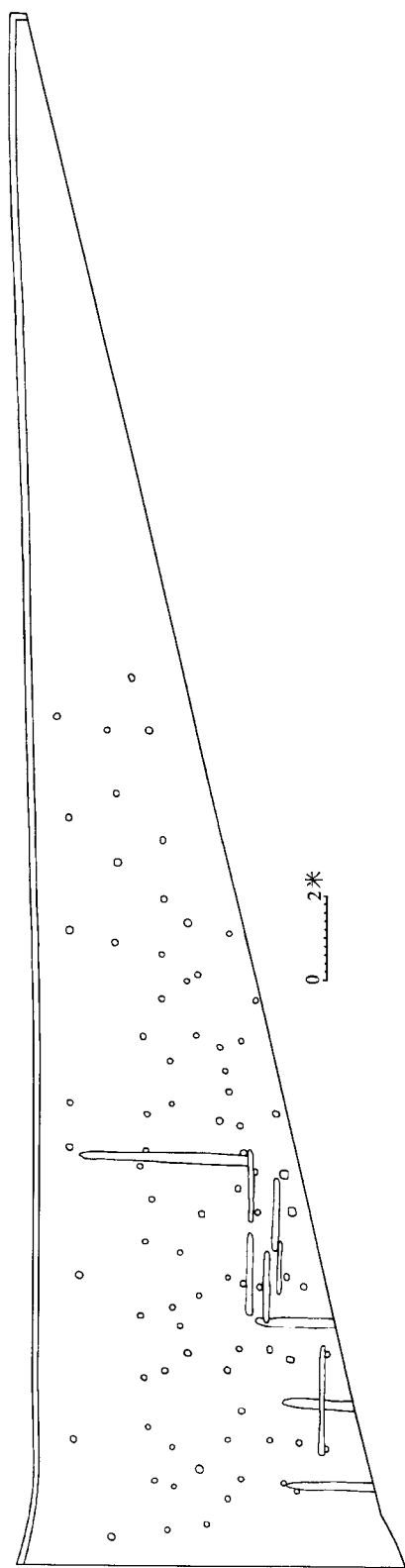
图 8A 墓道东壁内木筋分布示意图
