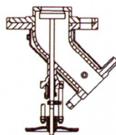
夹套下展式釜底放料阀 Jacket Down Side Discharging Valve
