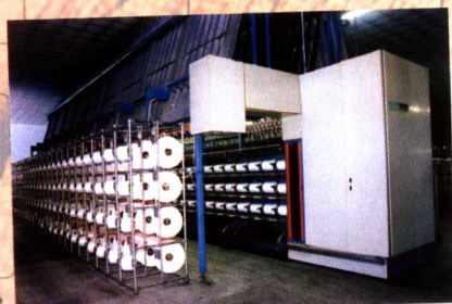
JWFK6-10 型、FK6-12 型、FK6-900 型假捻变形丝机
