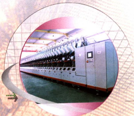
K2551 帘子线直捻机
