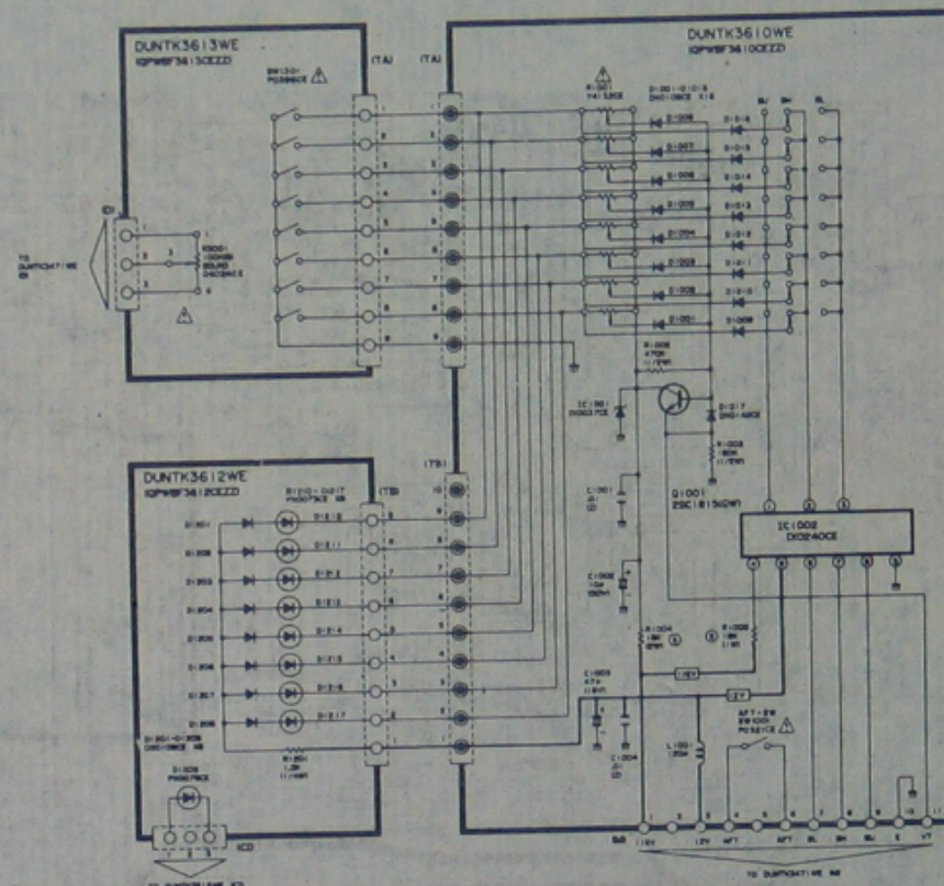
C-1405 预调器电路板
