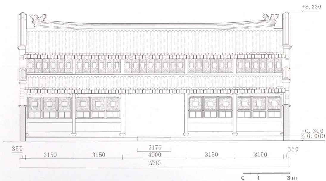
玉海楼前楼正立面图
