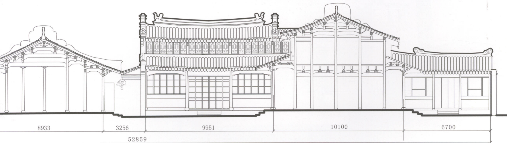
玉海楼总横剖面图
