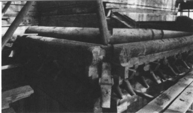
角楼抱厦大木结构
