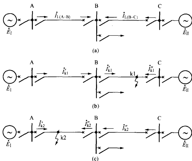
图 1.2 双侧电源网络接线
