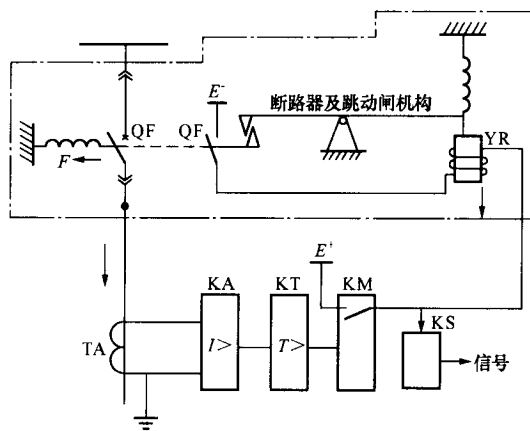
图 1.4 过电流保护工作原理图
