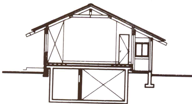
剖面图
