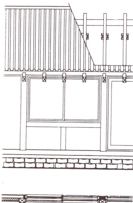
立面详细图
