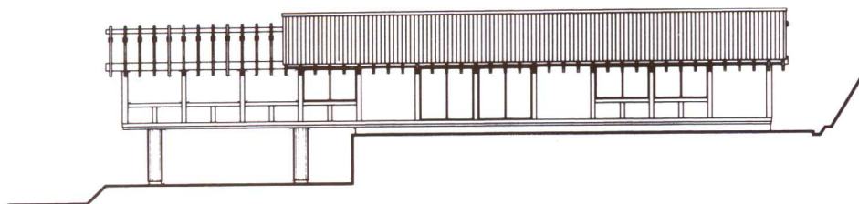
南侧立面图
