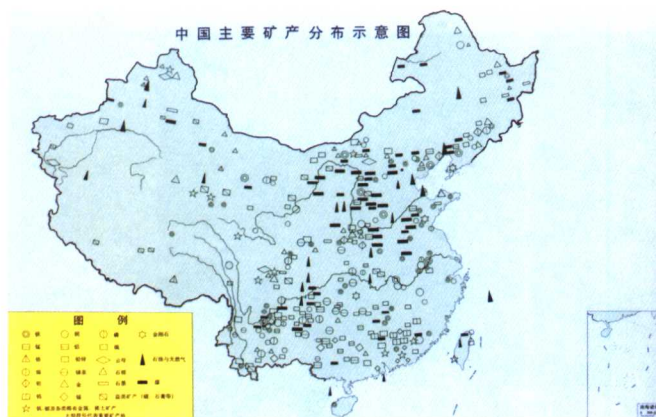
● 中国主要矿产分布示意图
