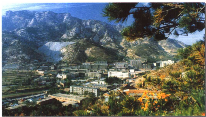
● 山东玲珑金矿
