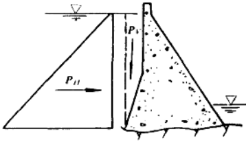
图 2-3 坝面静水压力计算图
