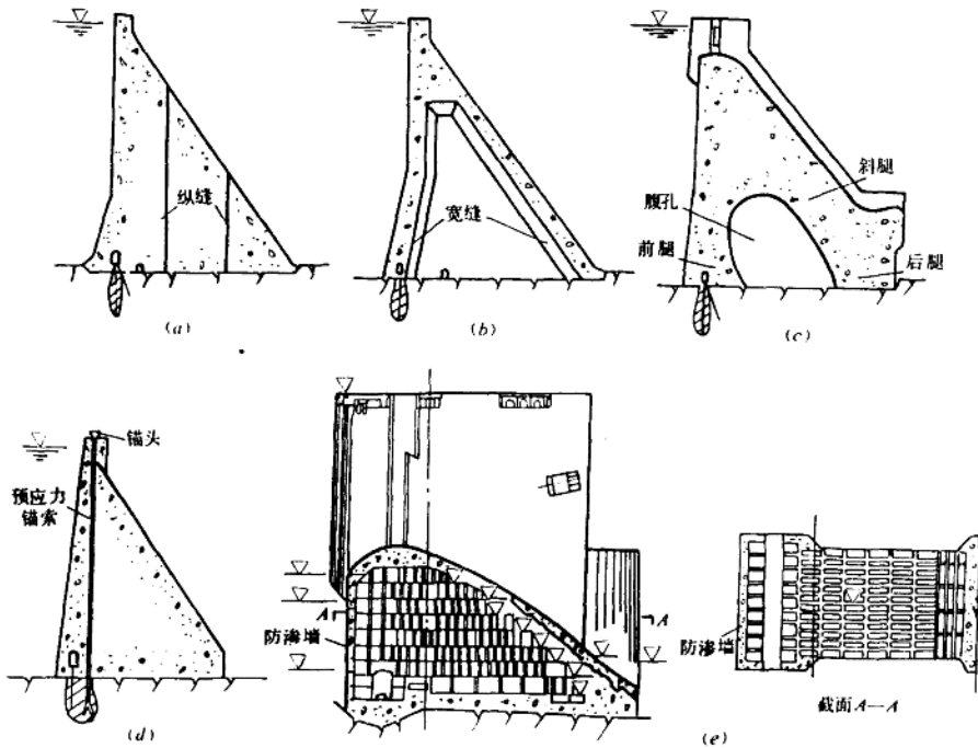
图 2-2 重力坝的型式
