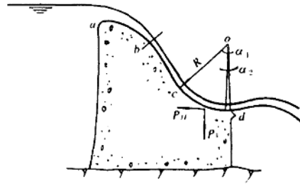
图 2-4 动水压力计算图
