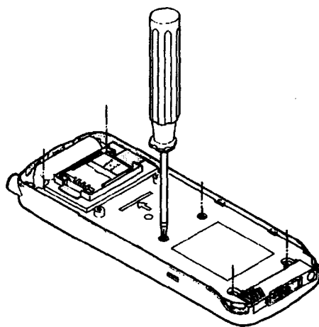
图 2-5 取下 6 个底板螺丝
