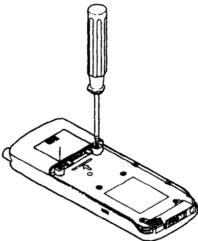
图 2-4 拧下背盖上的螺丝后打开背盖
