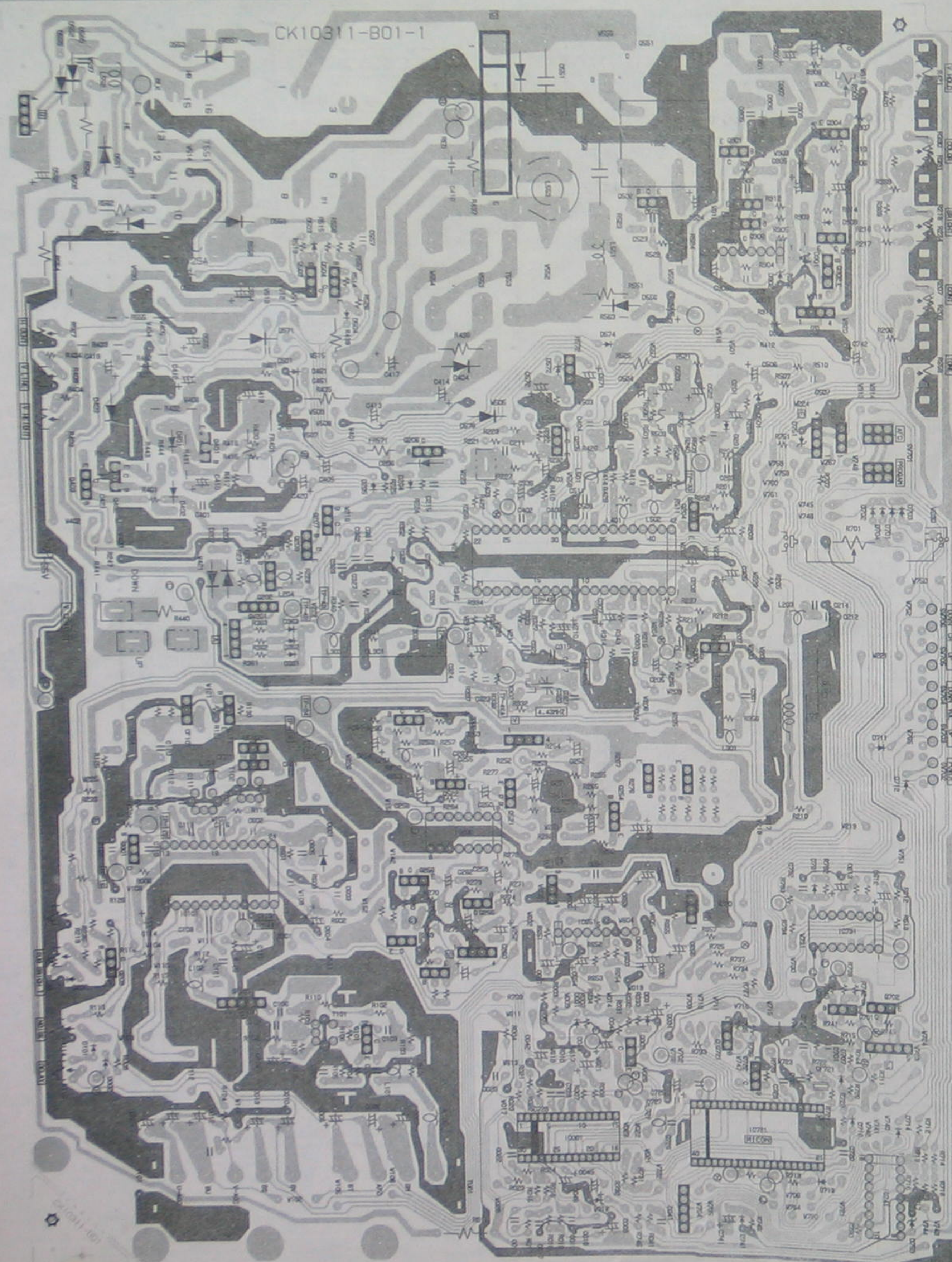
印制电路板图
