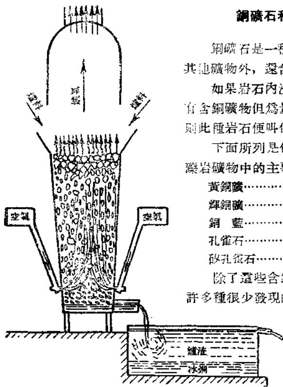
圖 2 鼓風爐斷面簡圖
