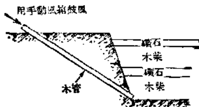
圖 1 坑法煉銅簡圖（垂直斷面）
